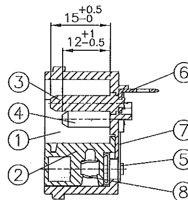
A-A 剖面
