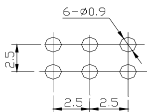
P.C.B HOLE DETAIL
