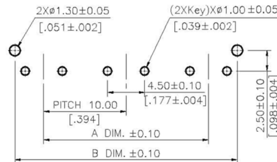
P.C.B. LAYOUT 3:1
